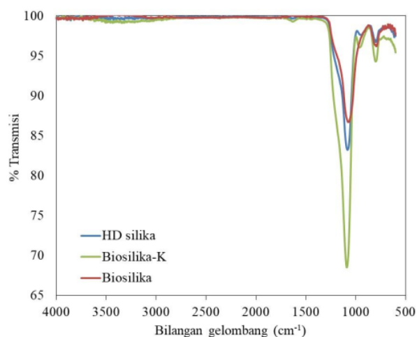
Gambar 1. Spektrum ATR-FTIR dari HD silika, biosilika B100-K dan B100
