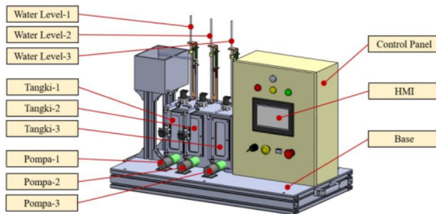
Gambar 3. Desain mekanik prototipe
