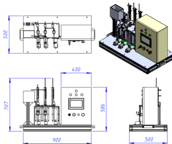
Gambar 4. Dimensi desain mekanik
