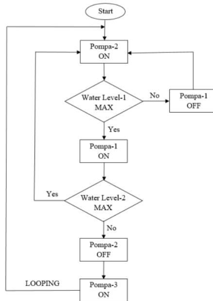
Gambar 8. Flowchart kinerja prototipe
