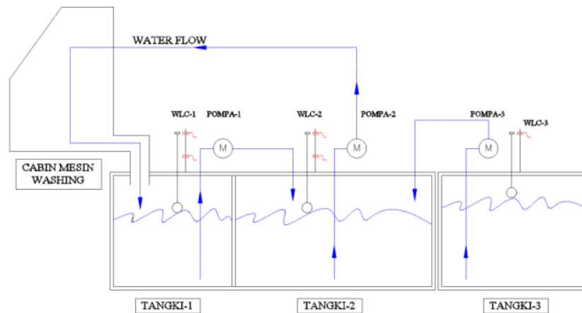
Gambar 2. Prototipe washer dengan sistem tiga tangki
