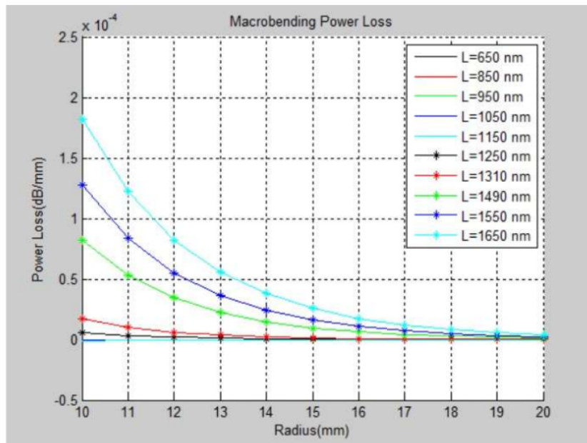
■ Gambar 7. Hasil simulasi macrobending pada pemrograman Matlab.
