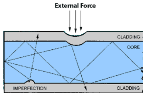
■ Gambar 3. Microbending yang diakibatkan oleh deformasi mikroskopik [15]
