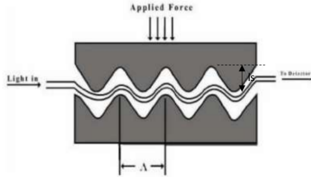
■ Gambar 5. Mekanisme uji microbending [22]
